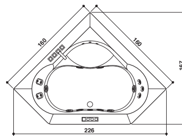
Double seat - Zwei Sitzflächen
